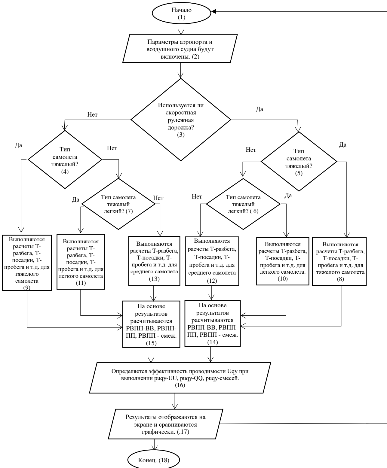
Рисунок 2. Алгоритм повышения пропускной способности взлетно-посадочной полосы аэродрома
